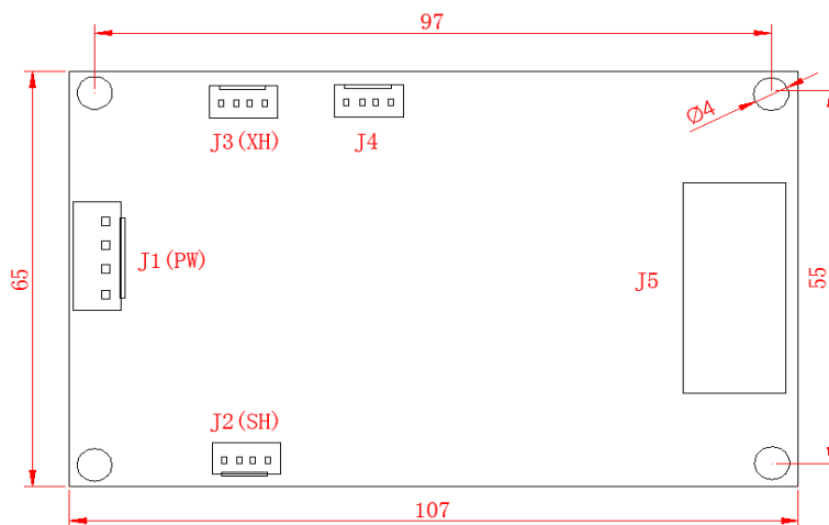
图 2.3 BL2000-HXJ-V9 尺寸图 (单位 mm)
