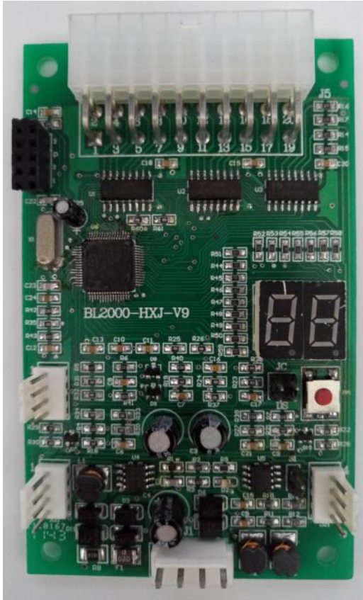
图 2.1 BL2000-HXJ-V9 实物图
